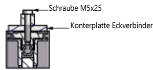
Schnitt C-C
