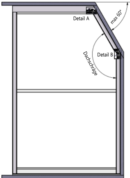
Schnitt C-C
